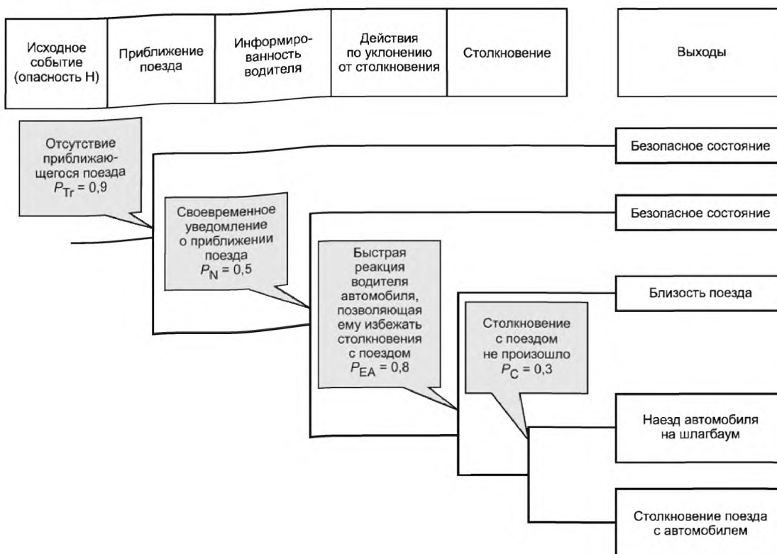
Рисунок В.4 — ETA для железнодорожного переезда
