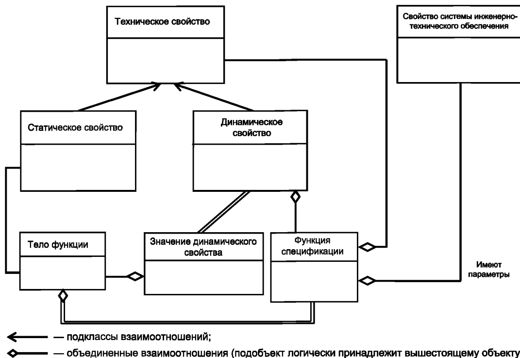
Рисунок 10 — Динамические свойства
