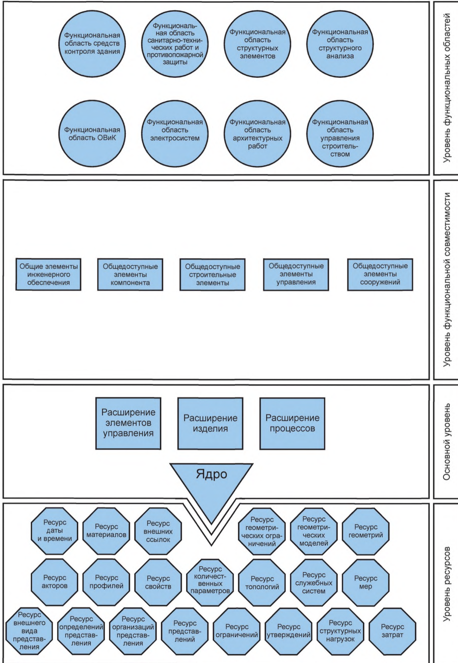
Рисунок 1 — Архитектура схемы данных с понятийными уровнями
