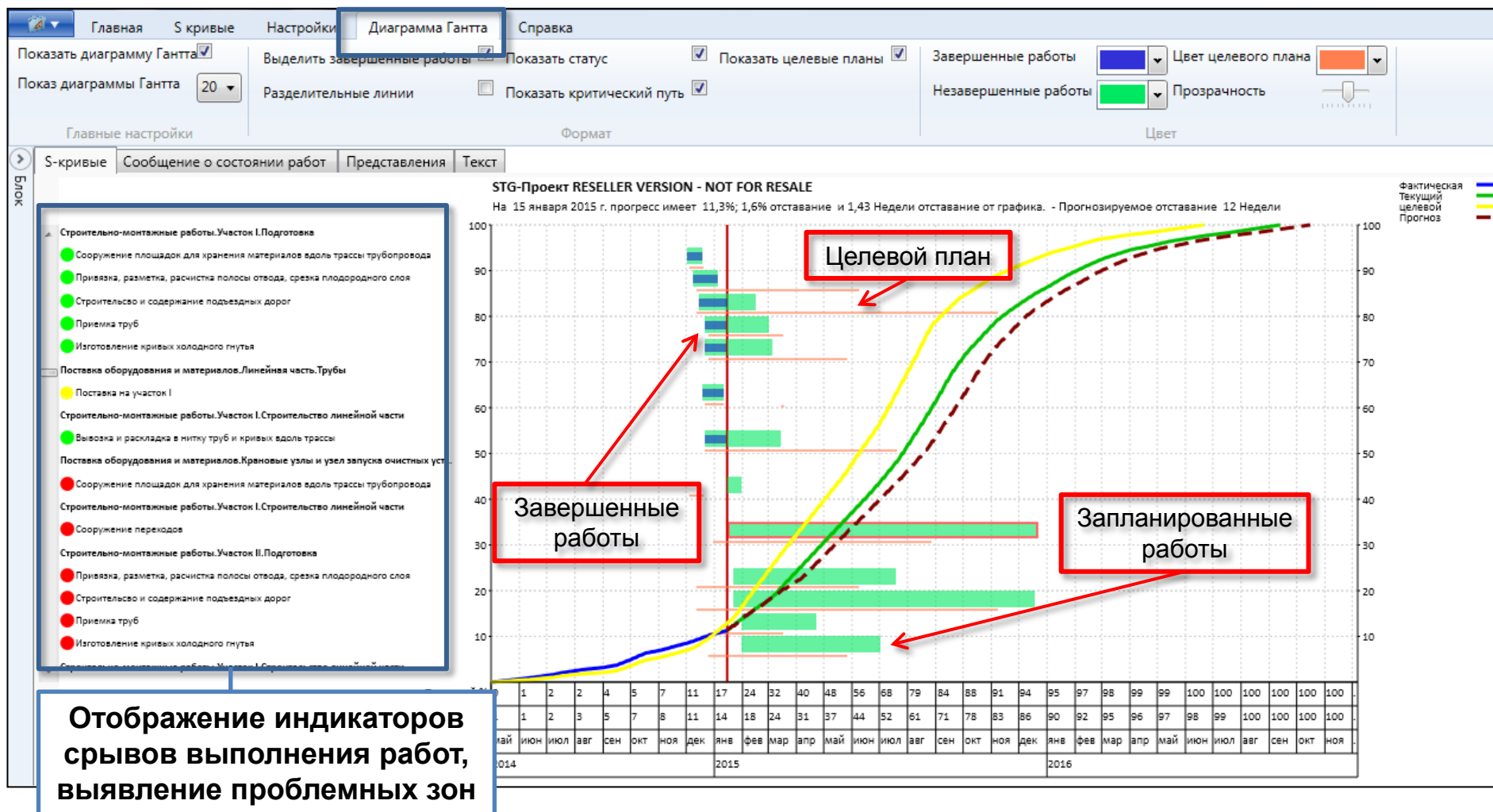
Совмещение Диаграммы Ганта и S-кривой
